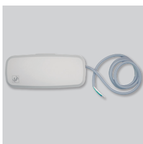
SPCM-WS ECOWATT PLUS como accesorio Permite conectar el ventilador a un smartphone y configurar el ventilador desde un entorno fácil e intuitivo, además de permitir ajustar parámetros avanzados.
