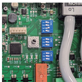
La ELECTRONICA ECOWATT PLUS permite ajustar parámetros y modificar modos de trabajo mediante potenciómetro y relés.
